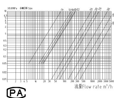
压力损失曲线
